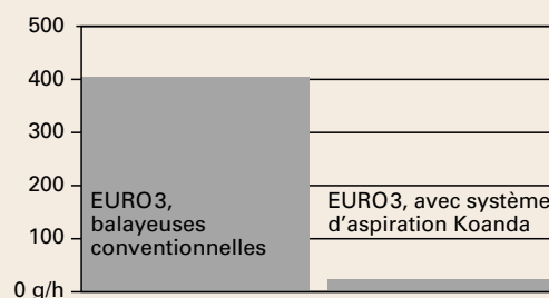
Rejet de particules des balayeuses
