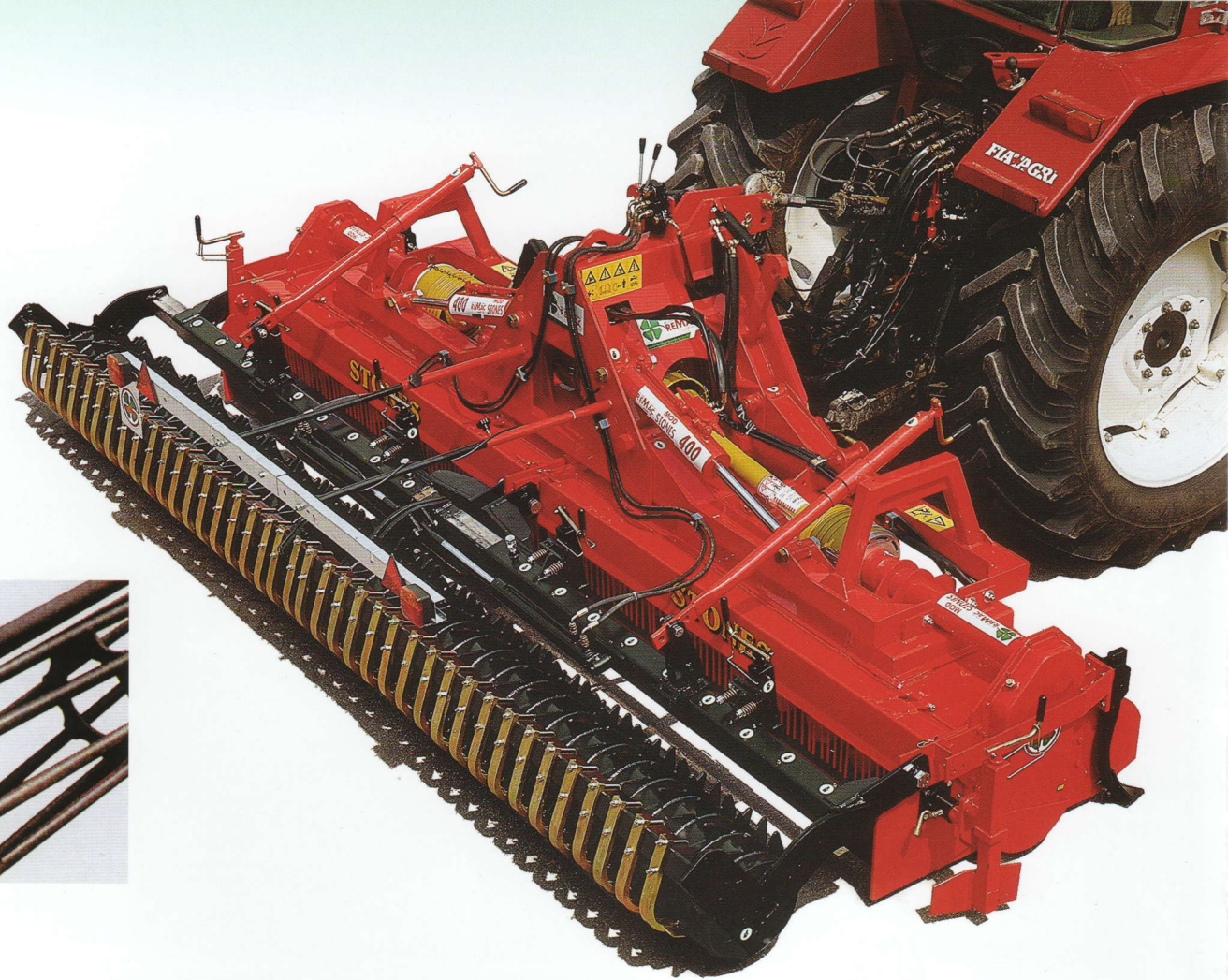
Preparazione del letto di semina per ortaggi in serra da metri 7,5. Seed-bed preparation for vegetables in green-houses 7.5 m width. Préparation du lit de semilles pour produits potagers de serre de 7,5 mètres. Saatbeet-Vorbereitung für Gemüse im Gewächshaus bis zu 7,5 m Arbeitsbreite.
