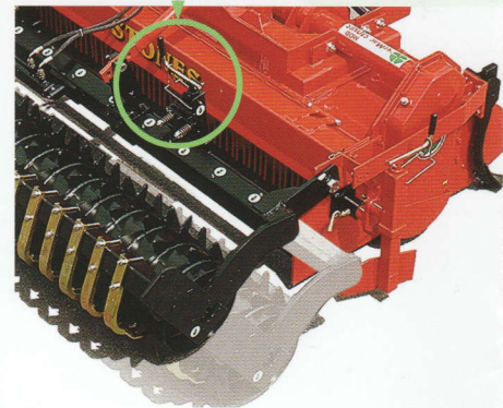
Spostamento idraulico del rullo. Hydraulic roller shifting. Déplacement hydraulique du rouleau. Hydraulisches Heben der Walzen.
