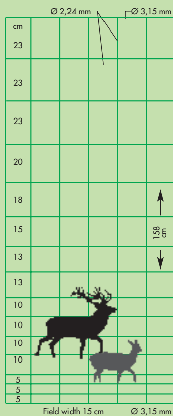
ProFORST-M/200 Height 200 cm / 16 fields ord.-no. 49002
