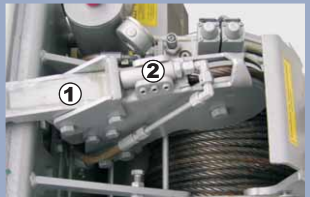
Oben: Hauptwelle mit Lamellenpaket Mitte: Antriebsstrang für höchste Kraftübertragung Unten: Seilverteilung ① mit Seileinlaufbremse ② a. W.
