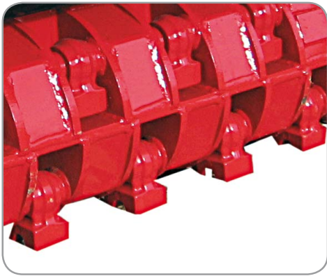
MIDIPIERRE rotor cu ciocane pendulare
